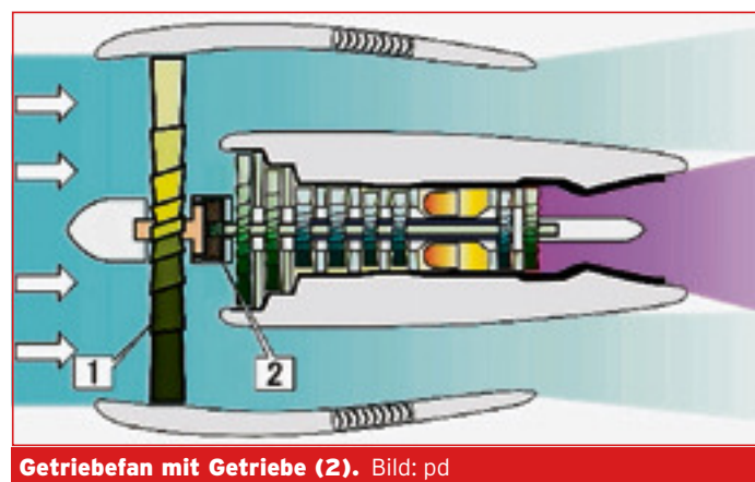
Getriebefan mit Getriebe (2). Bild: pd
